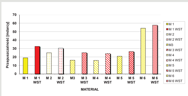
Rys. 10. Przepuszczalność badanych materiałów przed zastosowaniem 10 wstrząsów powietrznych i po nich
