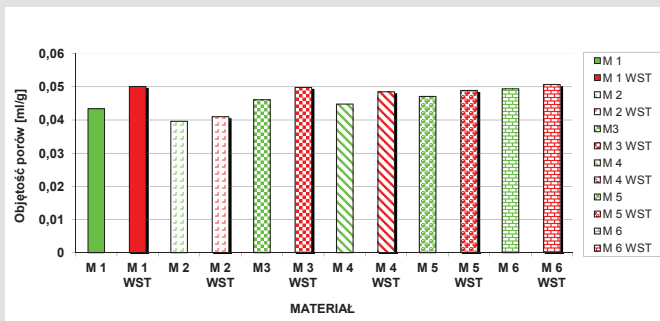
Rys. 4. Objętość porów w badanych materiałach przed zastosowaniem 10 wstrząsów powietrznych i po nich
