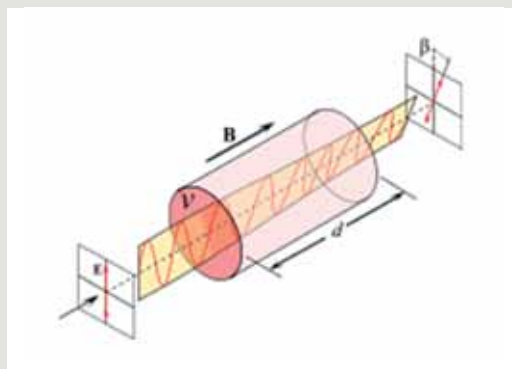
Rys. 1. Magnetoptyczny efekt Faraday'a.
