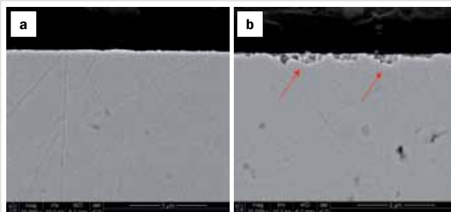
Rys. 4. Obrazy mikroskopowe próbek materiału OLD: a) przełamu próbki niestarzonej, b) przełamu próbki starzonej 5 godzin (pow. 20 000 \times ).
