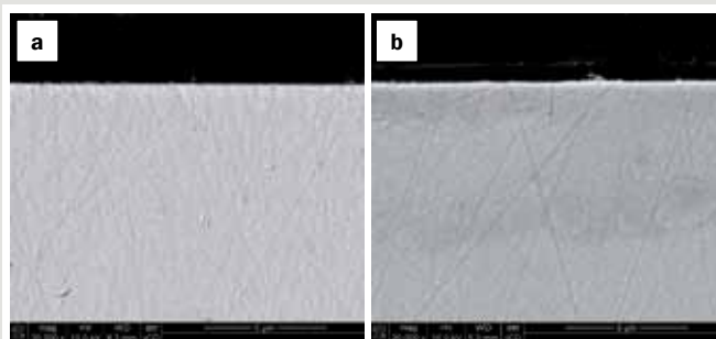
Rys. 5. Obrazy mikroskopowe próbek materiału SMILE: a) przełamu próbki niestarzonej, b) przełamu próbki starzonej 5 godzin (pow. 20 000 \times ).
