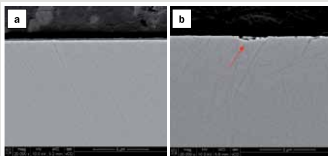
Rys. 3. Obrazy mikroskopowe próbek materiału HT: a) przełamu próbki niestarzonej, b) przełamu próbki starzonej 5 godzin (pow. 20 000 \times ).
